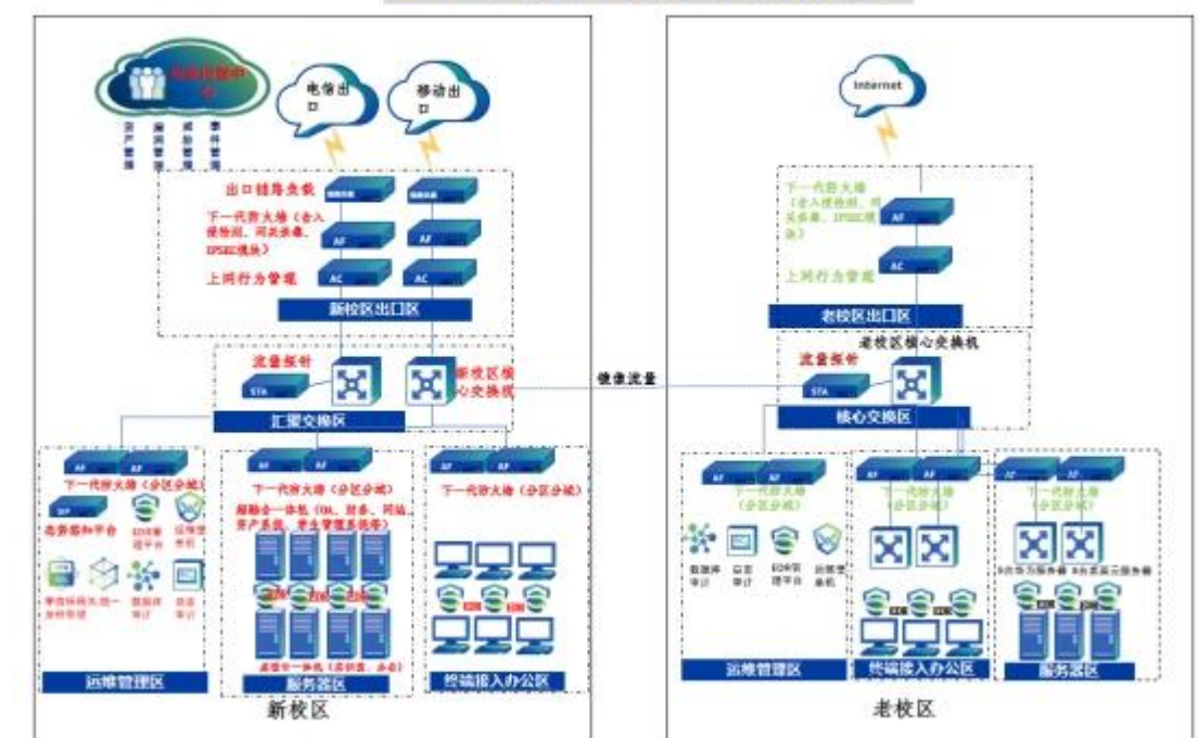
兰州外语职业学院网络拓扑规划
